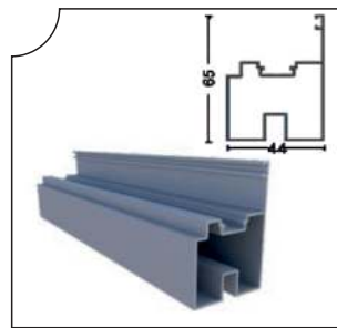
PRGLD-1008 8 mm İspanyolet Kol Profili 8 mm Espagnolette Arm Profile
