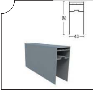
GLD-1005 Perdelik Ayar Profili Aluminum Curtain Profile Ağırlık/Weight 1.254 kg/m
