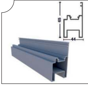
ISICM21-1009 İspanyolet Kollu Profil Espagnolette Arm Profile
