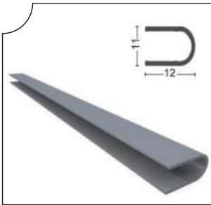
ALMFTL-1005 D Fıtıl Aluminum "D" Seal Ağırlık/Weight 0.140 kg/m
