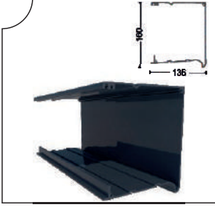
GYTN-1701 Üst Kutu Antrasit Gri Upper Box Anthracite Gray
