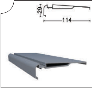
GYTN-1704 Küpeşte Profili Railing Profile
