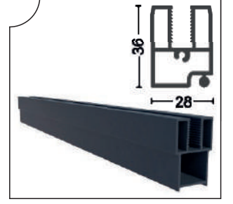
GYTN-1725 Dikey Baza 8 mm Vertical Base Ağırlık/Weight 0.706 kg/m
