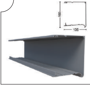
GYTN-1701 Üst Kutu Profili Upper Box Profile
