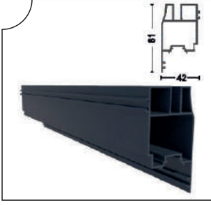
GYTN-1726 Ağırlır Kanat 8 mm Profile Of Opens 8 mm Ağırlık/Weight 1.14 kg/m
