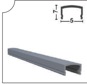
GYTN-1705 Küpeşte Çıtası Profili Railing Slat Profile
